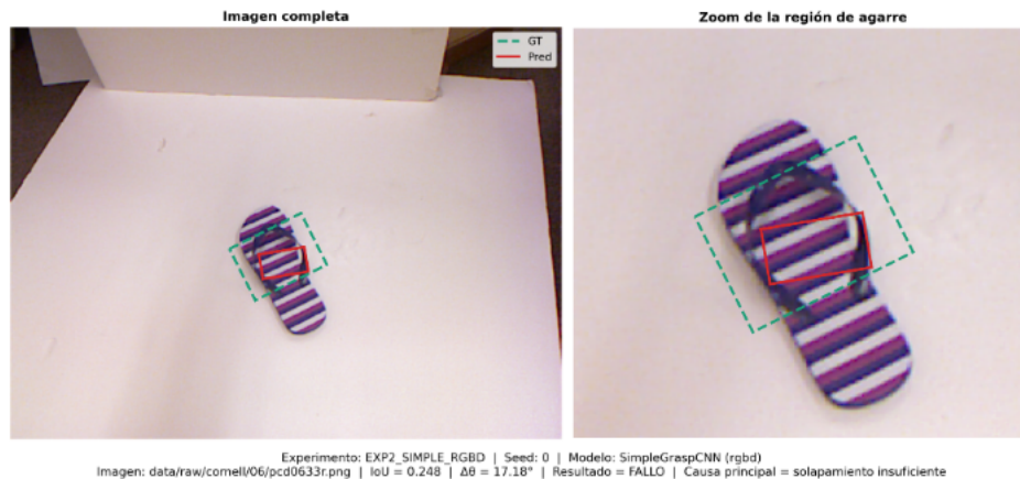
Ilustración 5-15. Caso límite de falso negativo por IoU insuficiente (EXP2_SIMPLE_RGBD, seed 0). La predicción mantiene una orientación compatible con la referencia ( \Delta\theta = 17,18^\circ ), pero no alcanza el umbral Cornell de solapamiento ( \text{IoU} = 0,248 < 0,25 ), por lo que se clasifica como fallo
